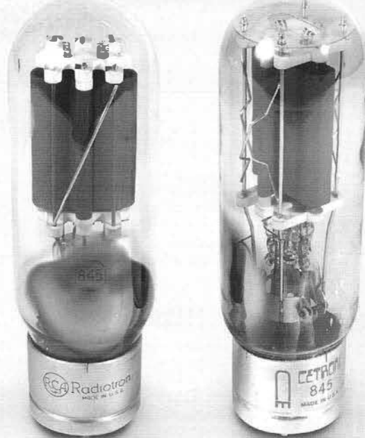
RCA 845 & CETRON 845
